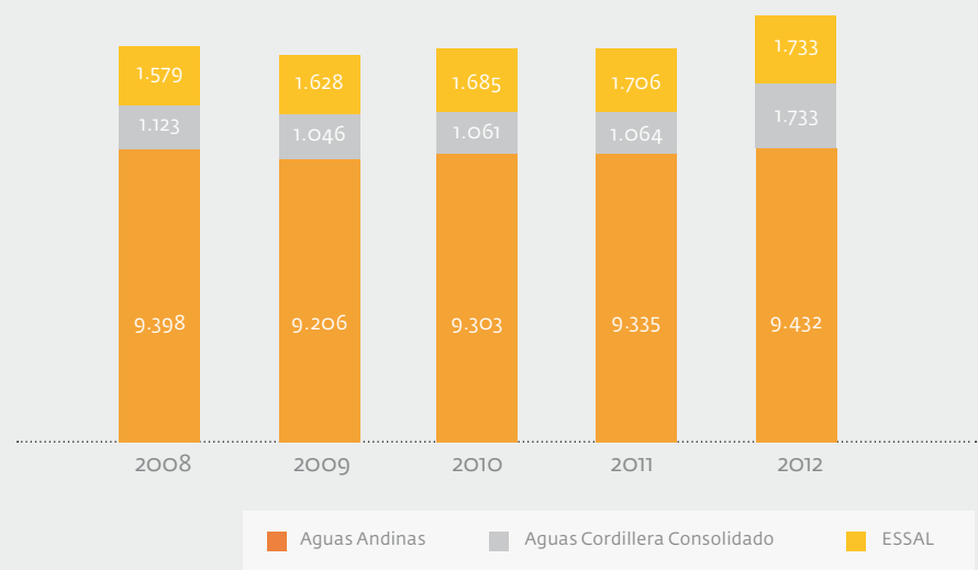
Gráfico N°12: Evolución longitud de la red de recolección consolidada de Aguas Andinas (kms) TRATAMIENTO Y DISPOSICIÓN DE AGUAS SERVIDAS
